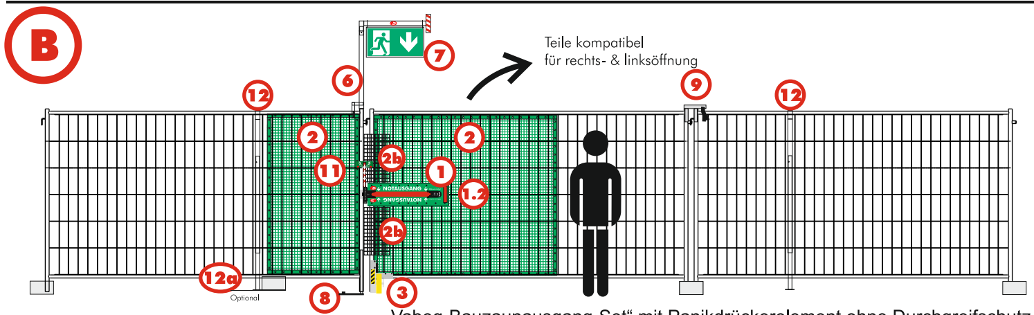
„Vabeg-Bauzaun-Ausgang-Set“ mit Panikdrückerelement ohne Durchgreifschutz Toröffnung in Fluchtrichtung nach rechts; Montage ebenso nach links öffnend möglich.
